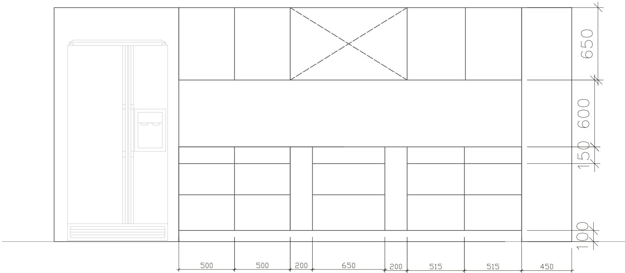
ELEVATION B
